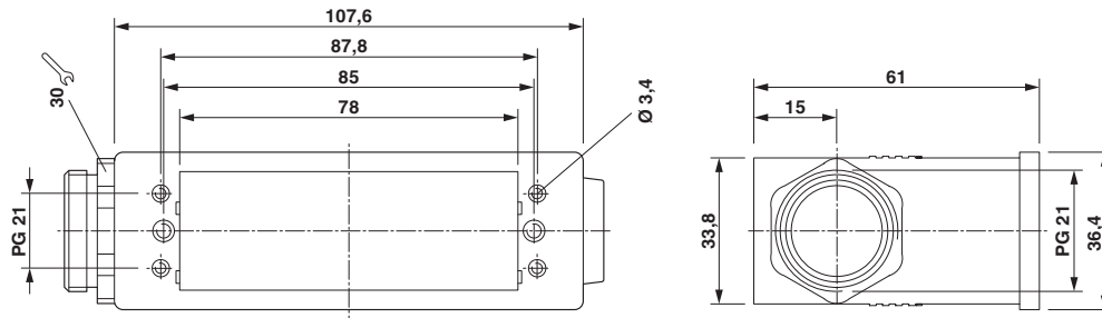
Esquema de dimensiones
