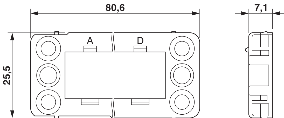
Esquema de dimensiones marco empotrado
