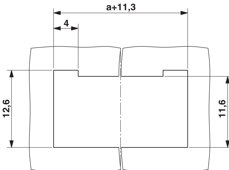
Plano esquemático
