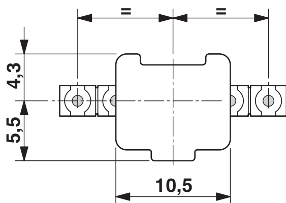
Esquema de dimensiones
