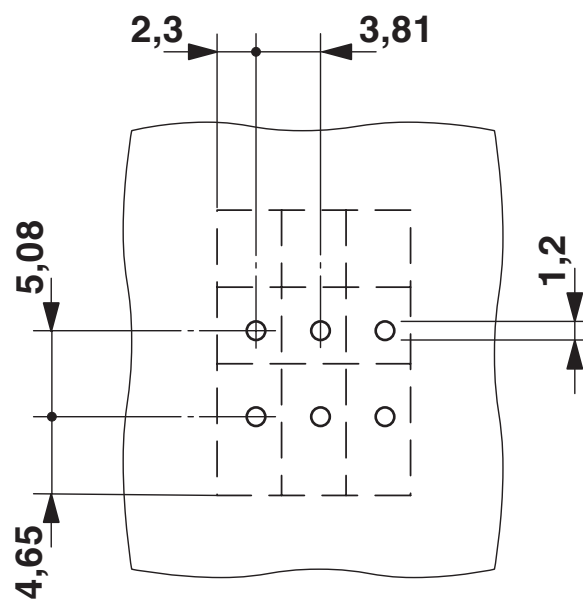
Esquema de taladros/geometría pads soldadura
