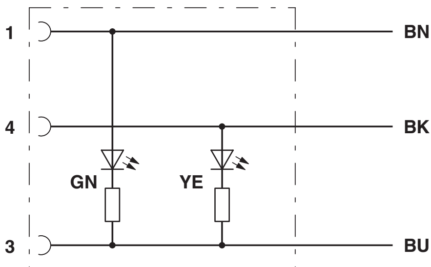
Diagrama eléctrico
