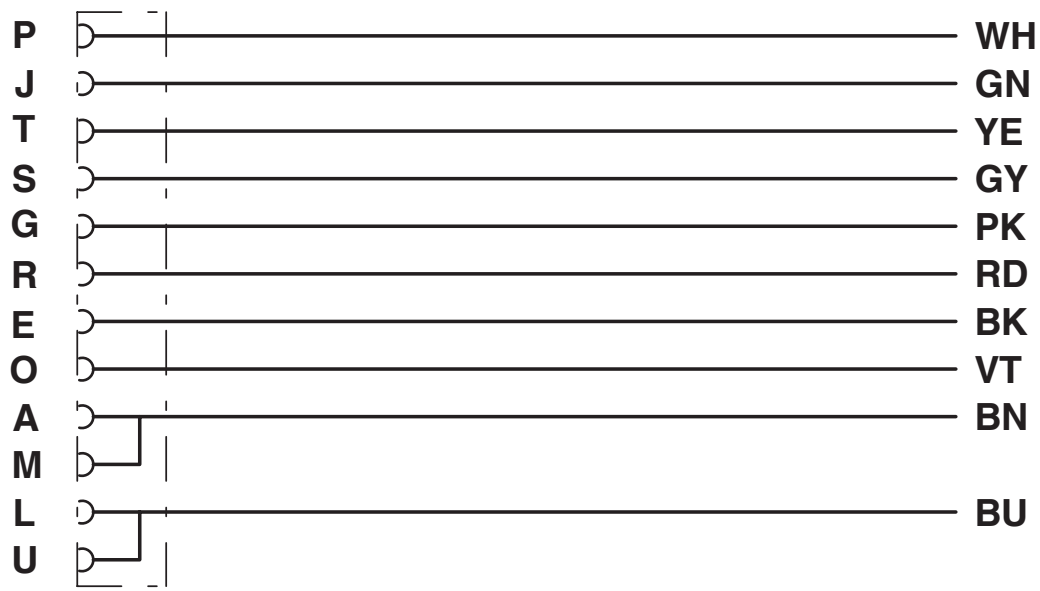
Ocupación de contactos del conector hembra M16
