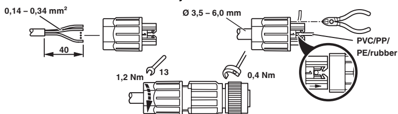
Dibujo funcional
