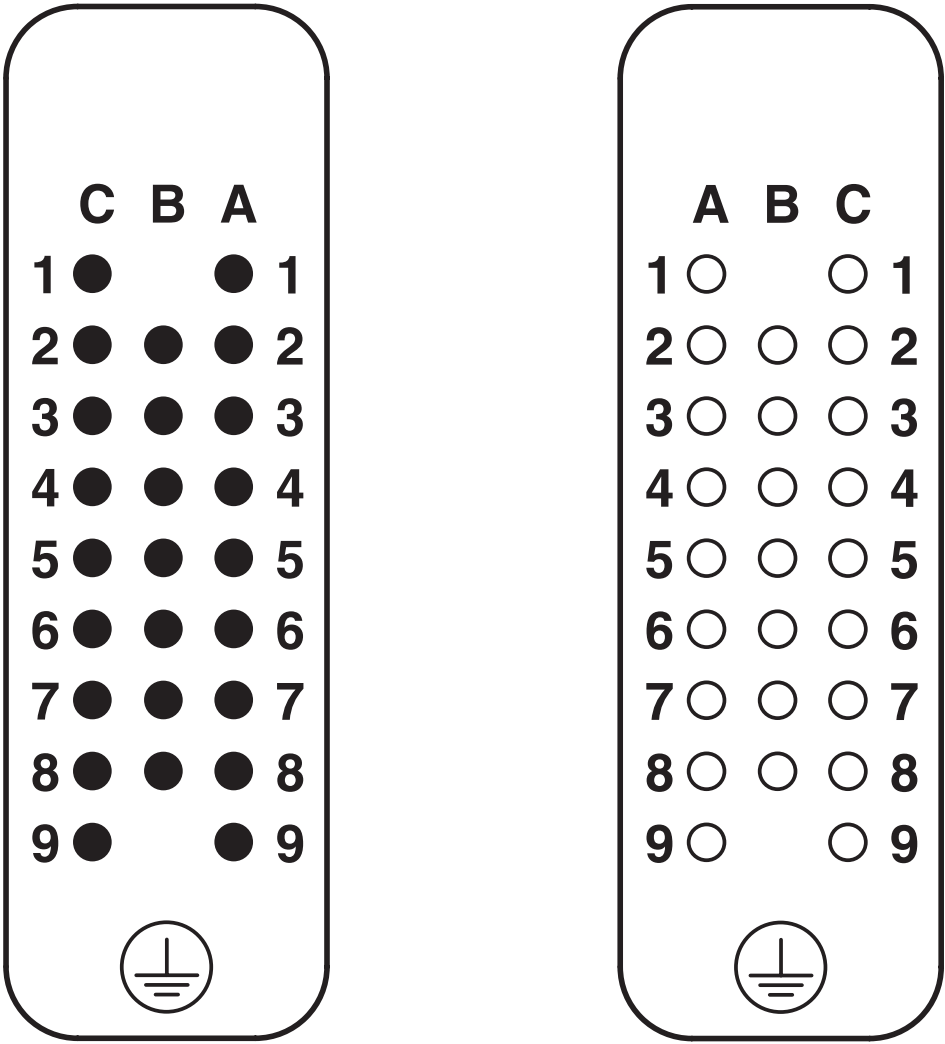
Plano esquemático
