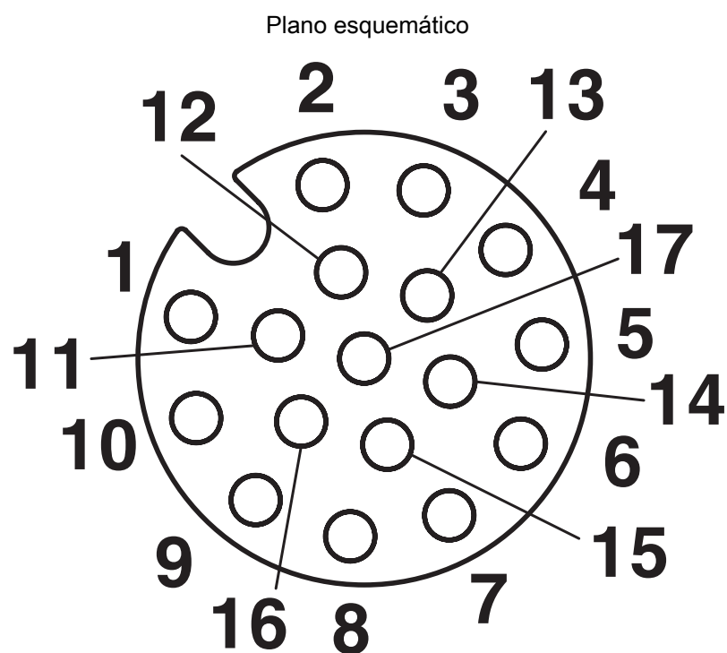
Esquema de polos del conector hembra M12, 17 polos, vista de la cara de hembras
