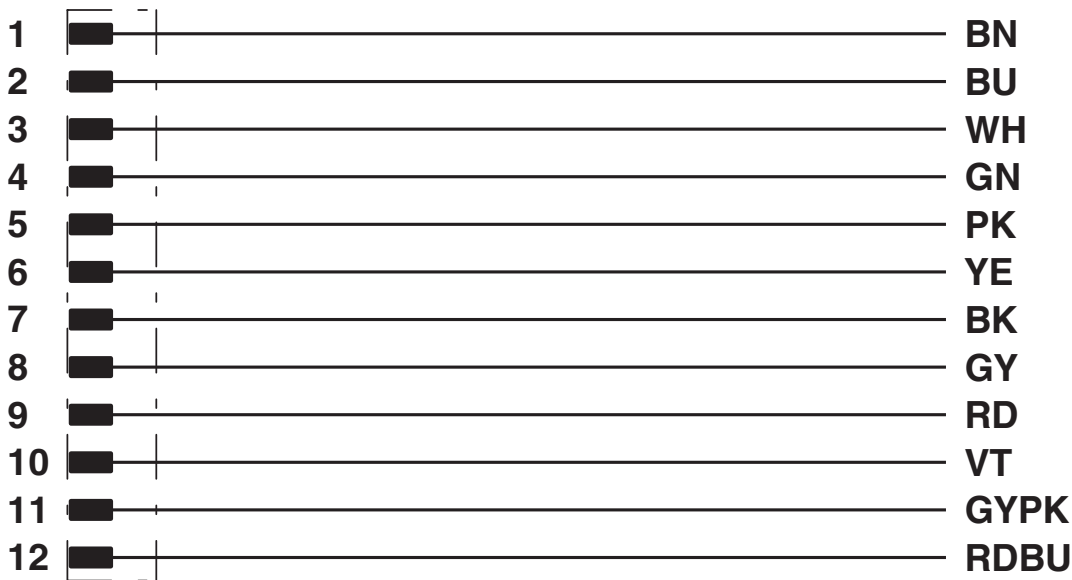
Diagrama eléctrico
