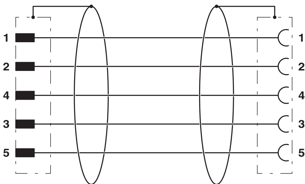
Diagrama eléctrico
