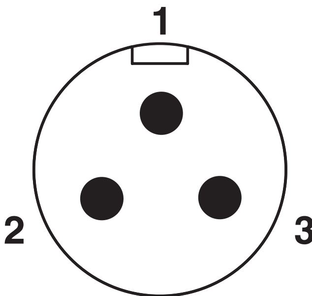
Plano esquemático
