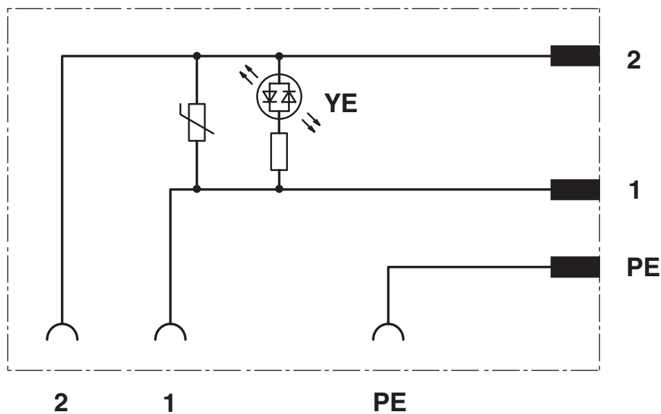
Diagrama eléctrico
