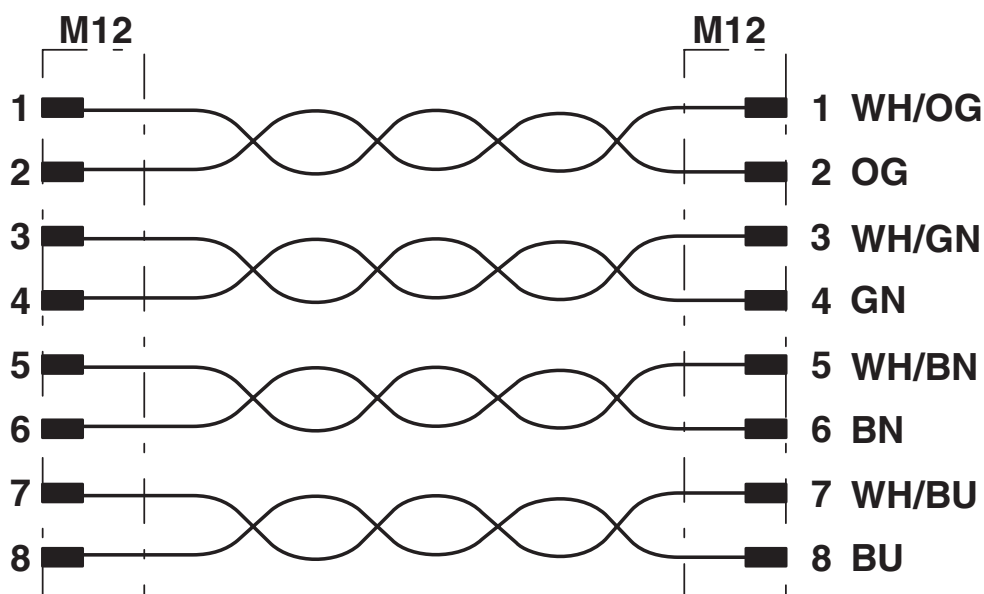
Ocupación de contactos de los machos M12
