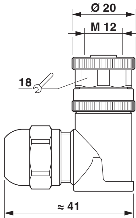
Esquema de dimensiones
