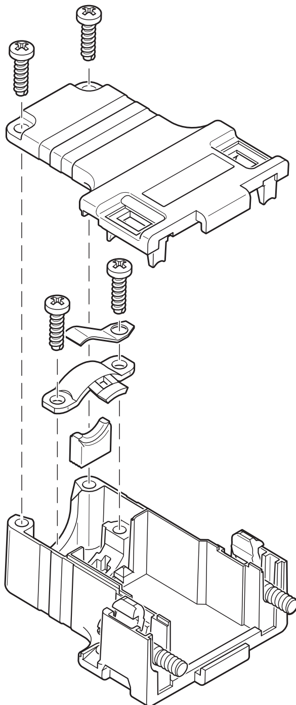
Plano esquemático
