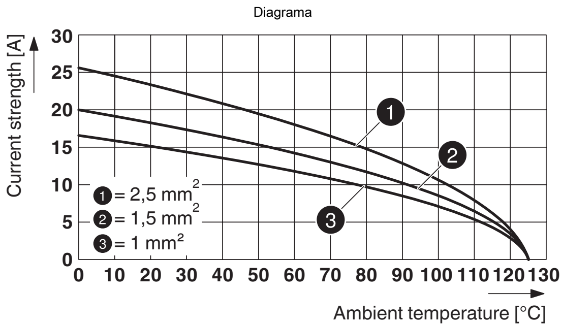
Diagrama derating (6 módulos en la carcasa HC-B 24)
