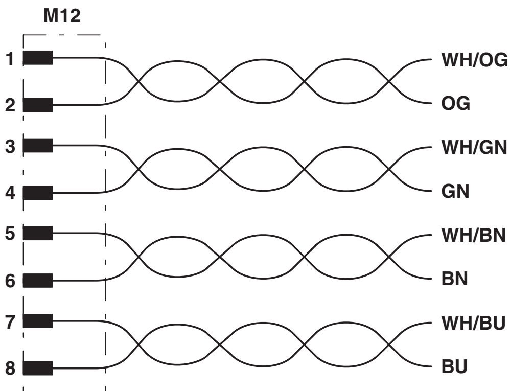
Diagrama eléctrico
