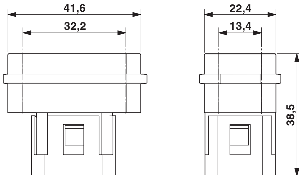
Esquema de dimensiones HC-COM-8-ESTC
