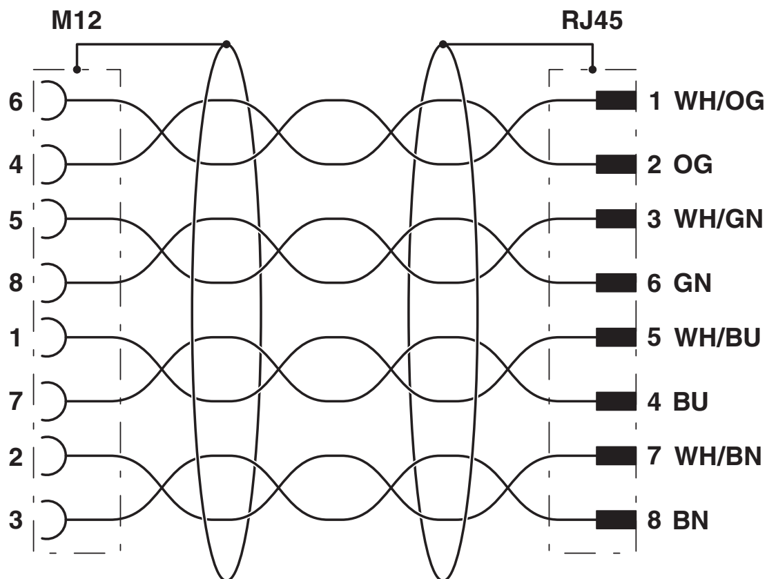
Diagrama eléctrico
