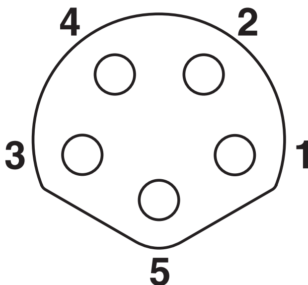
Esquema polos, lado de hembra conexión, M8, 5 polos, codificado B
