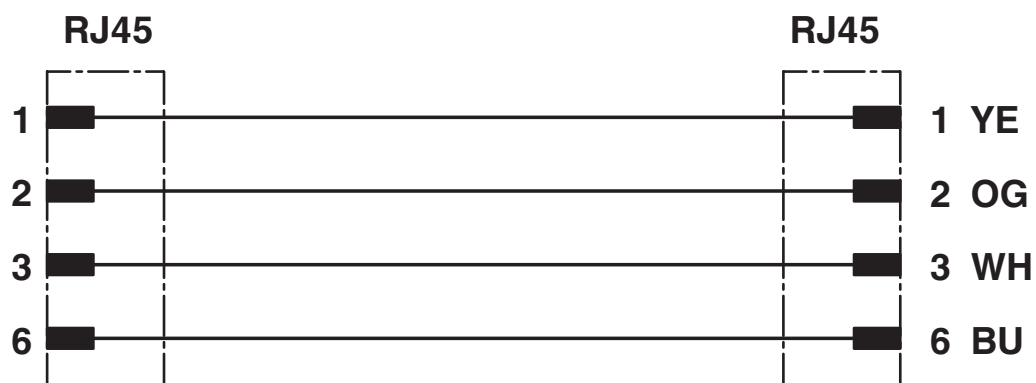
Diagrama eléctrico
