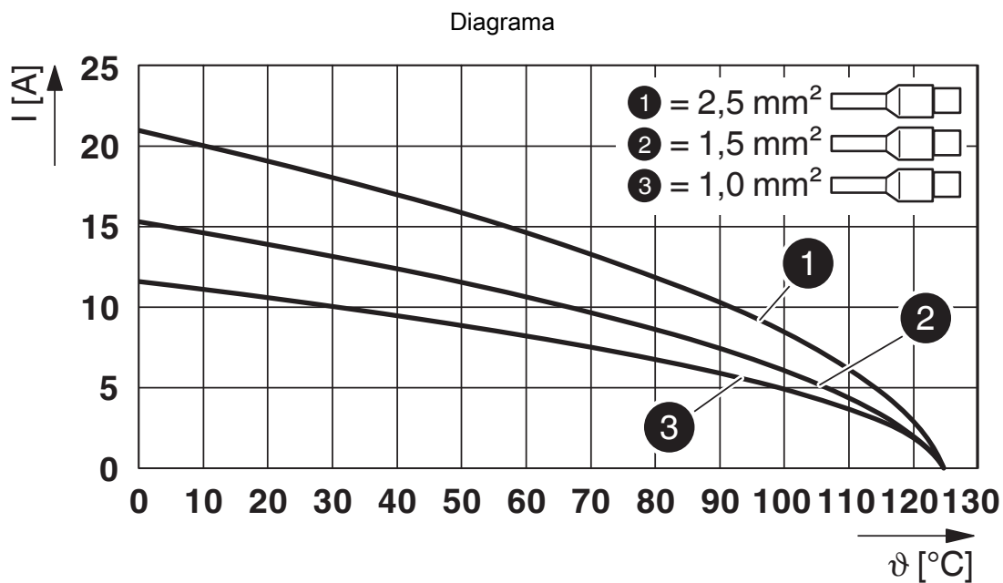
Diagrama derating para conductores flexibles con puntera
