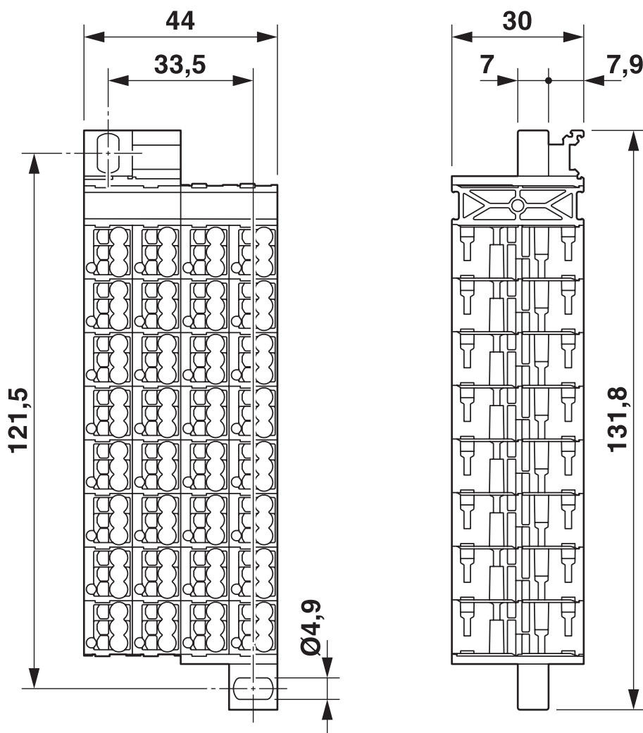
Maßzeichnung
