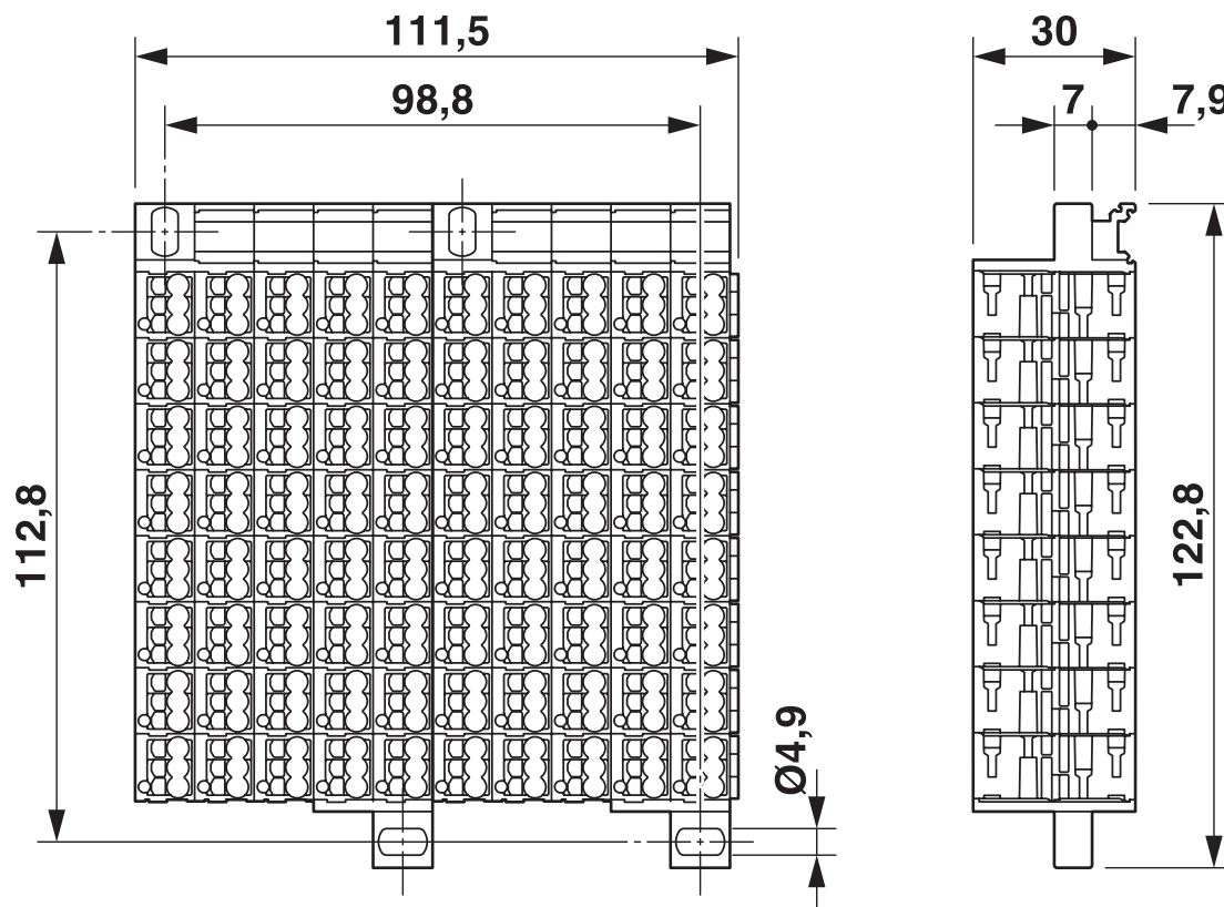
Maßzeichnung
