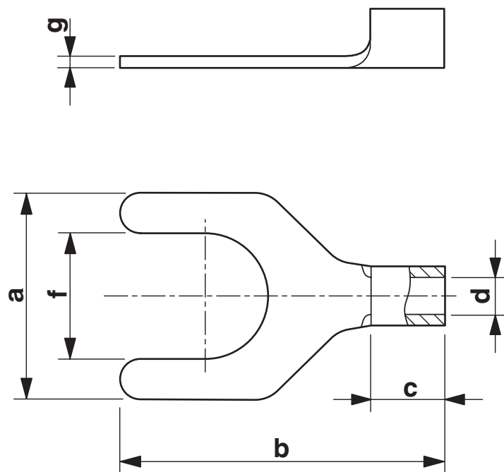
Maßzeichnung
