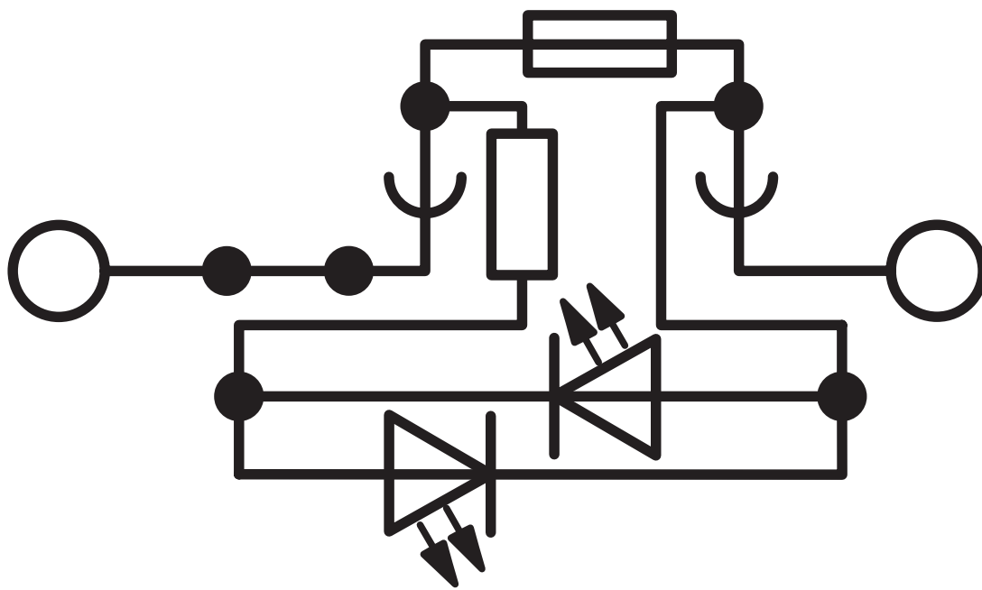
Schaltplan
