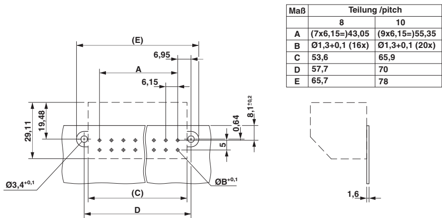
Maßzeichnung
