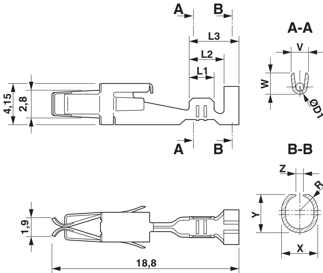
Maßzeichnung
