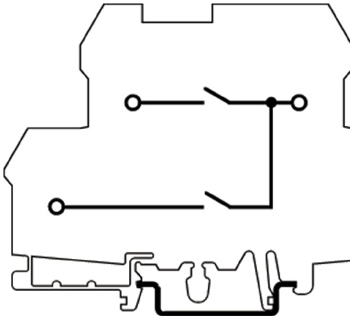
Schaltplan
