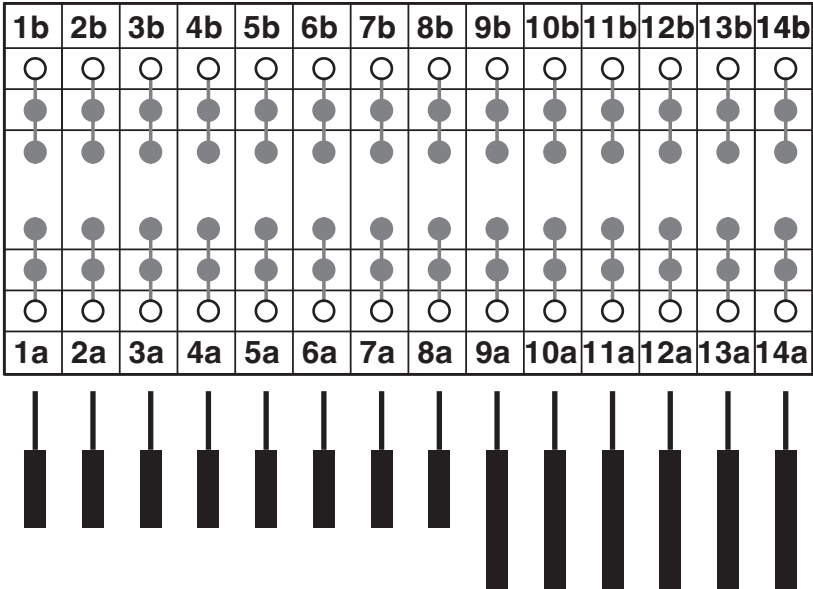
Schaltplan
