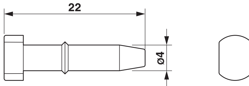
Maßzeichnung
