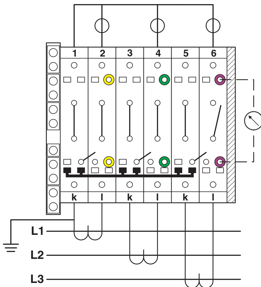
Anschlusszeichnung
