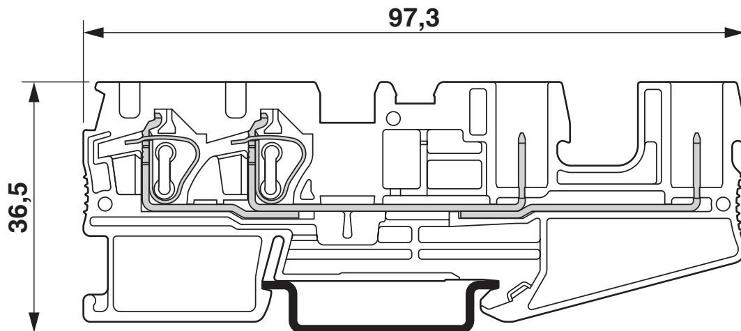
Maßzeichnung
