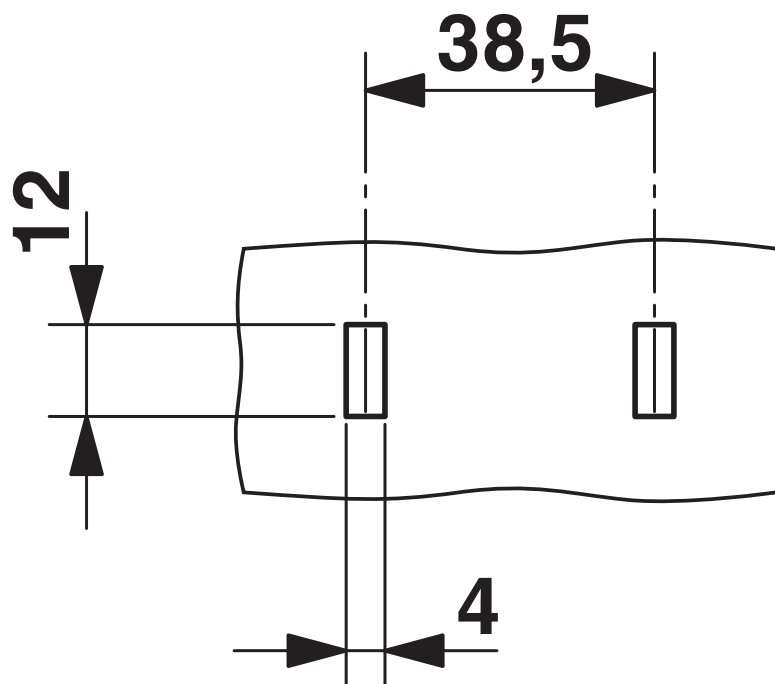
Maßzeichnung
