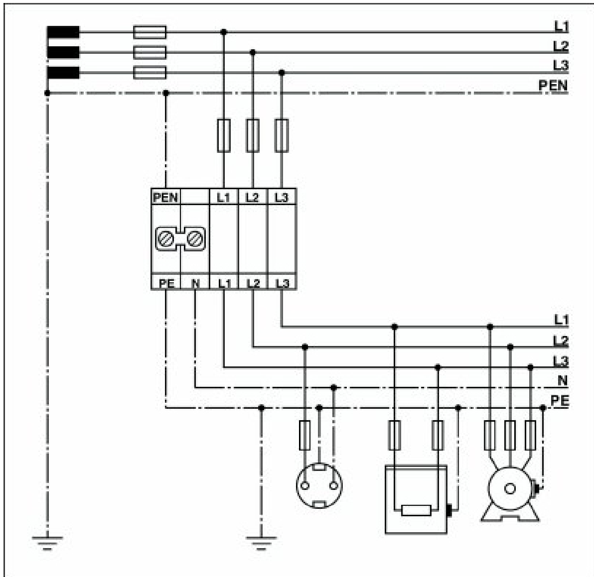
Anschlusszeichnung
