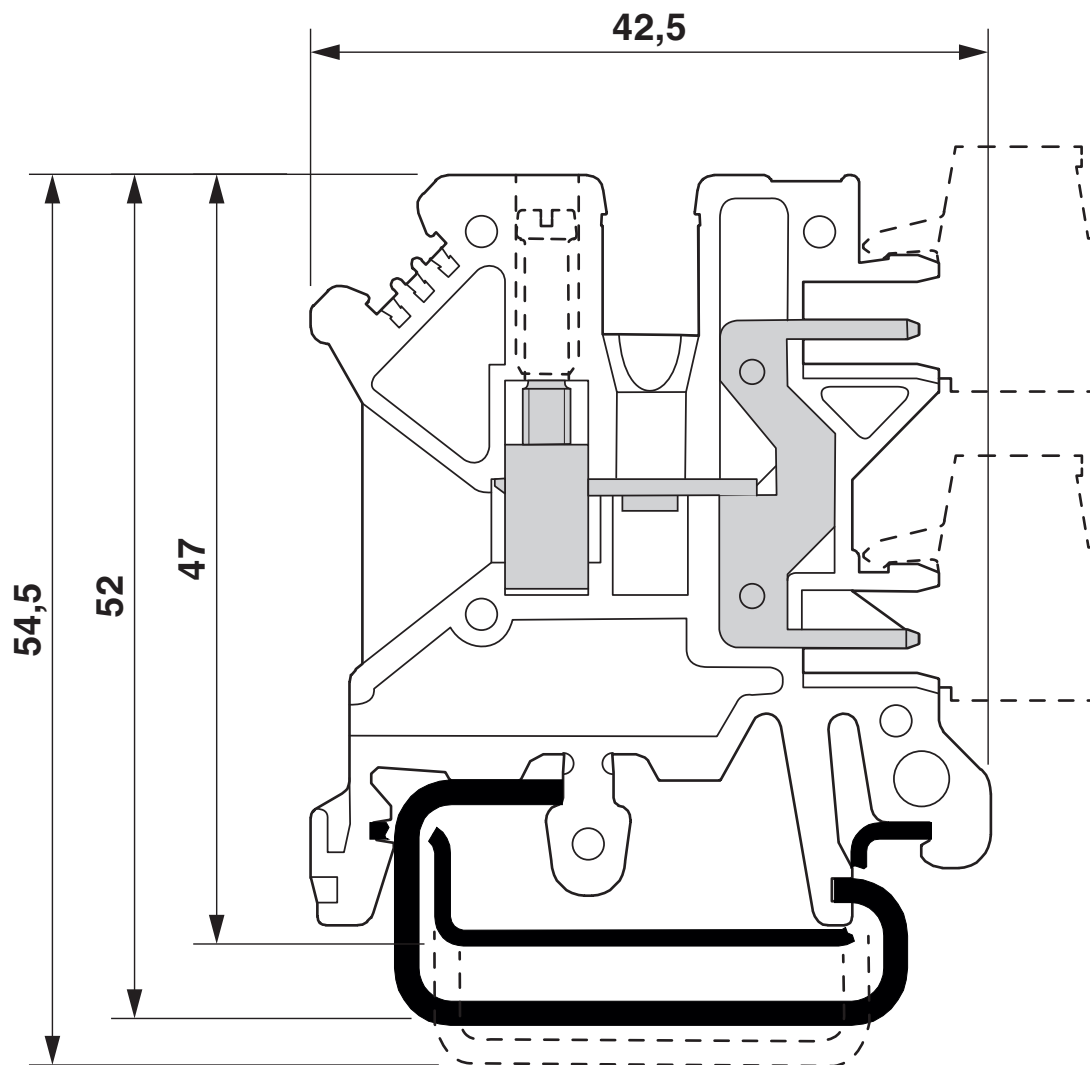
Maßzeichnung
