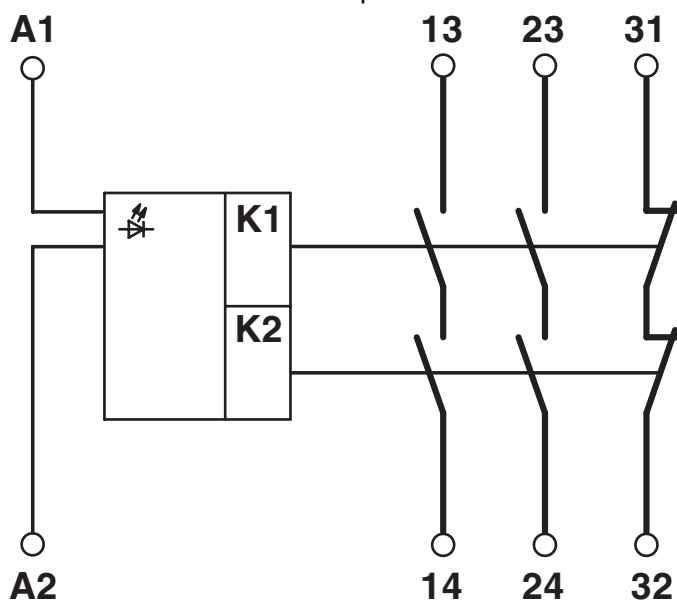
Schaltplan
