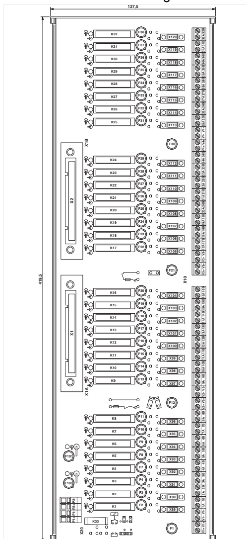
Maßzeichnung
