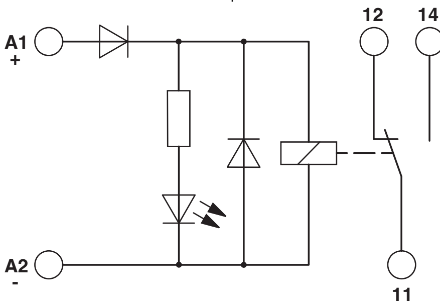
Schaltplan
