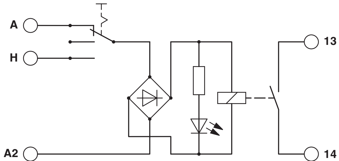
Schaltplan
