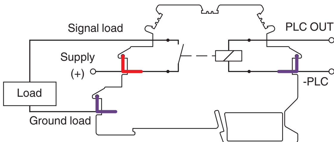
Anschlussbelegung DEK-REL-...AKT
