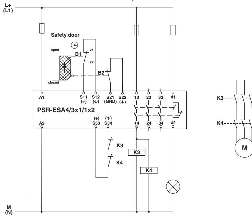
Schaltplan
