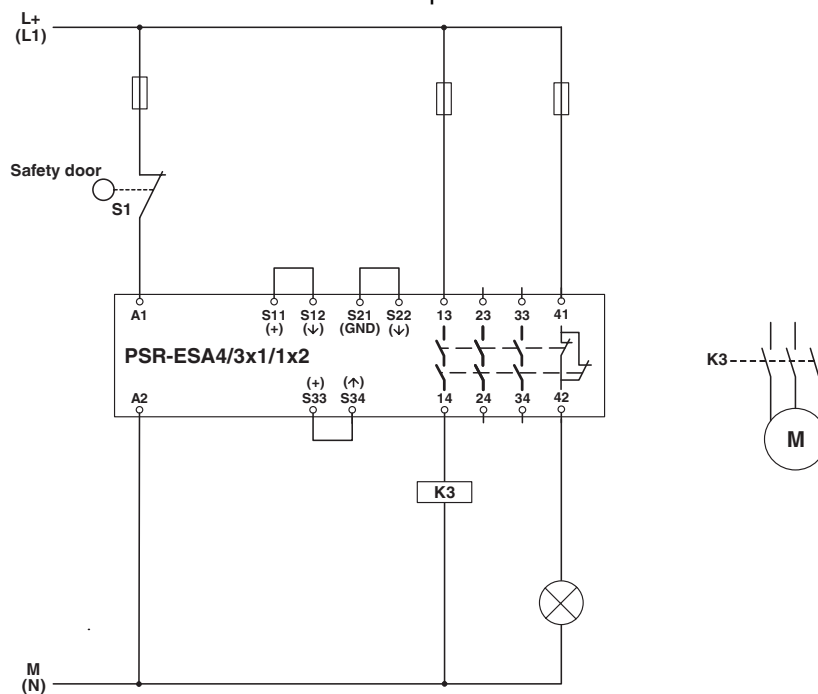
Schaltplan
