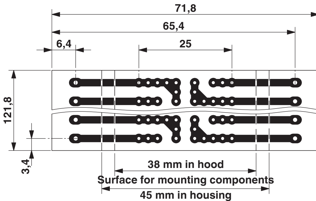
Maßzeichnung
