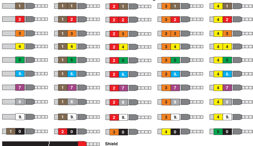
Schemazeichnung
