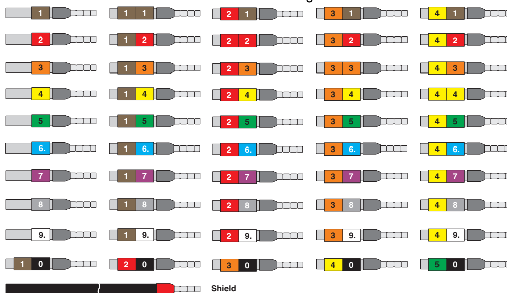
Schemazeichnung
