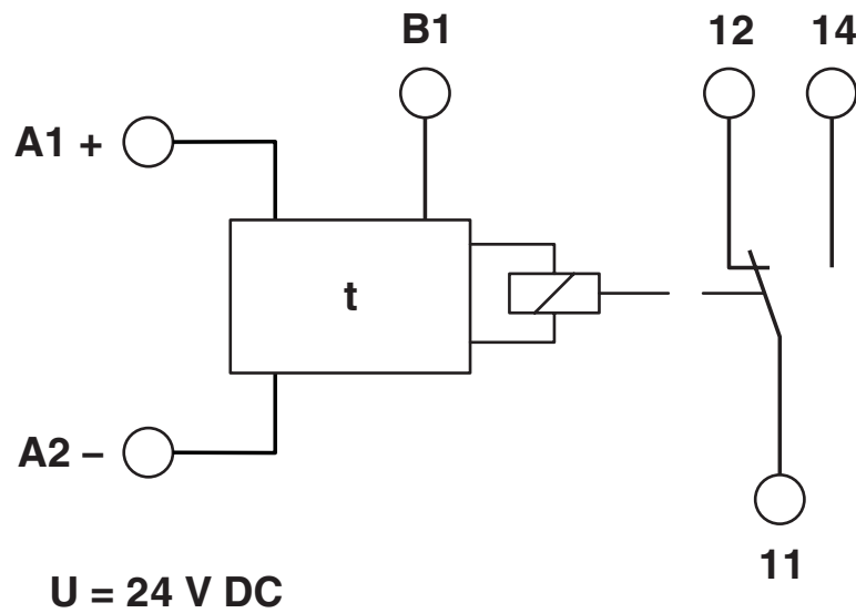
Blockschaltbild
