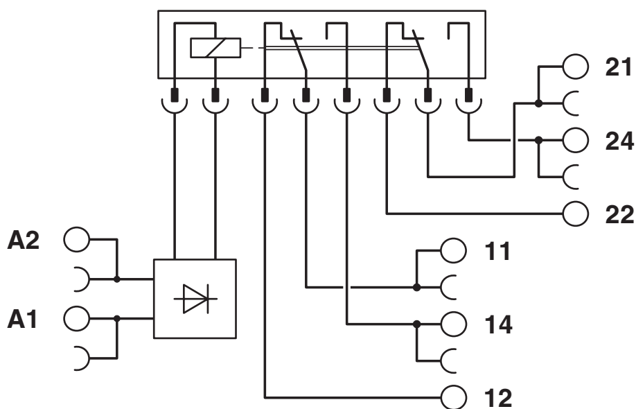
Schaltplan
