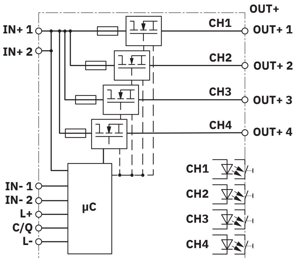
Blockschaltbild
